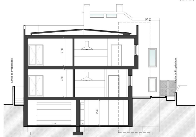
CORTE 4
