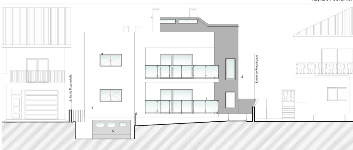
ALÇADO PRINCIPAL
