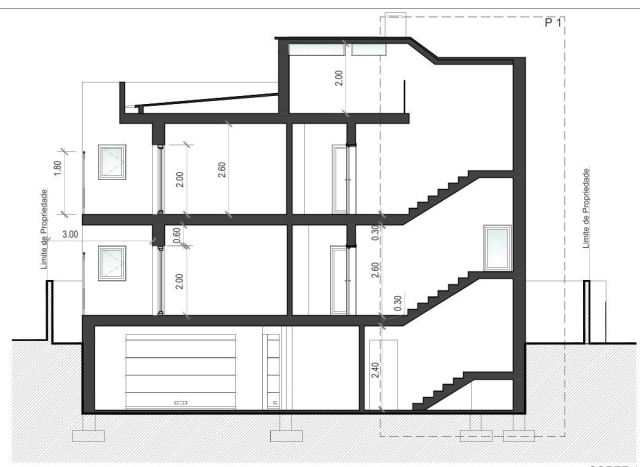
CORTE 1
