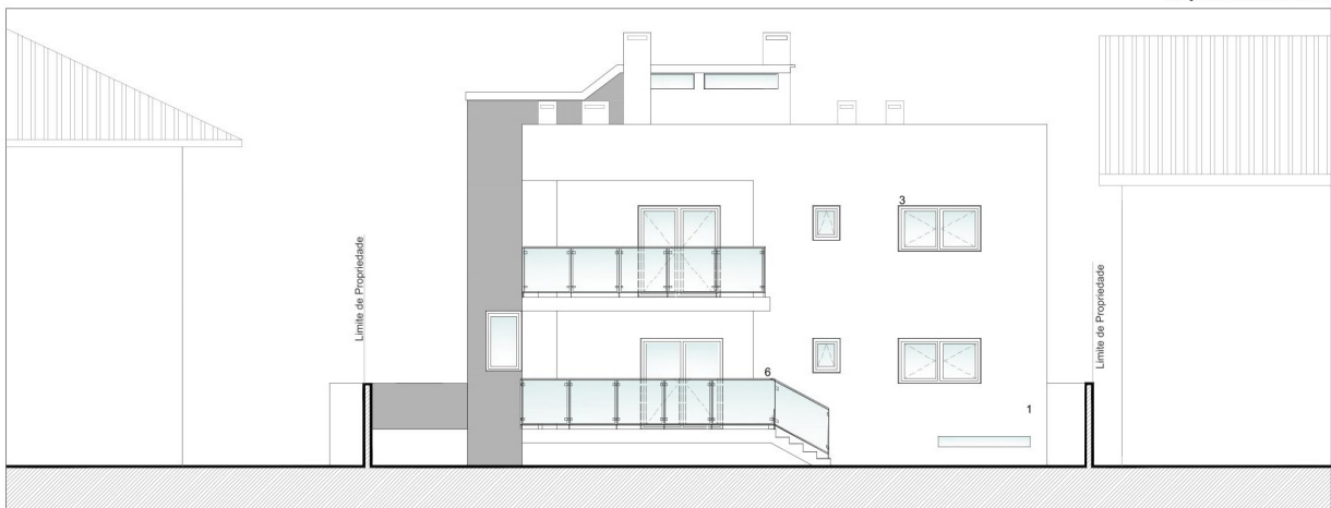
ALÇADO POSTERIOR
