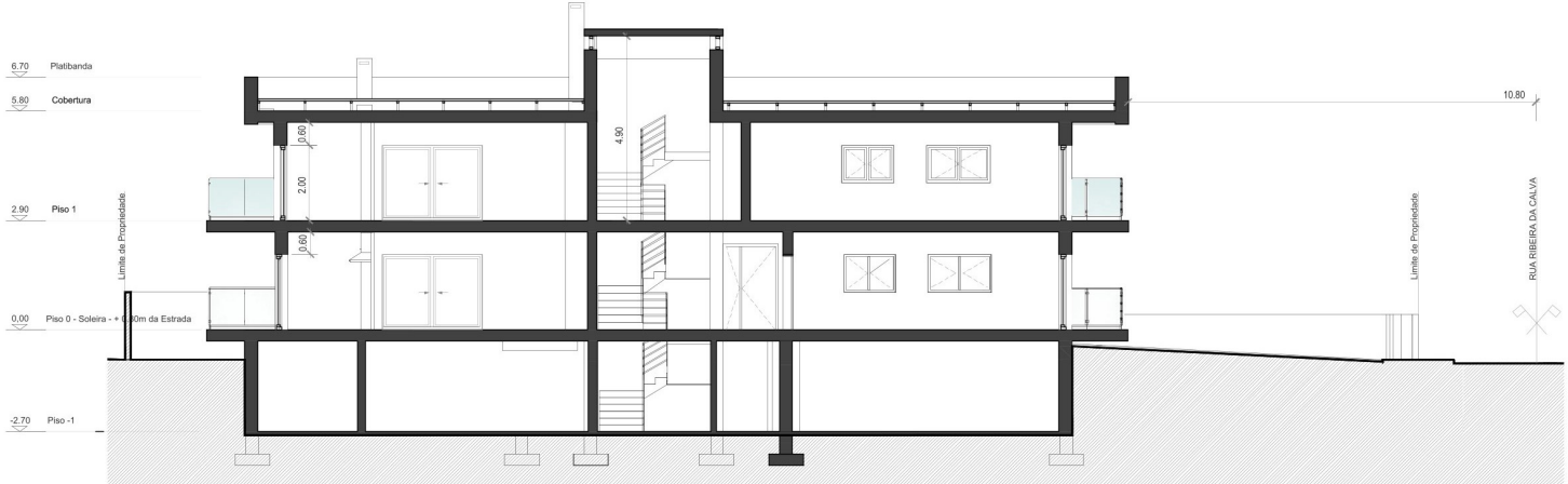
CORTE 2
