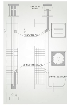
VENTILAÇÃO FORÇADA
