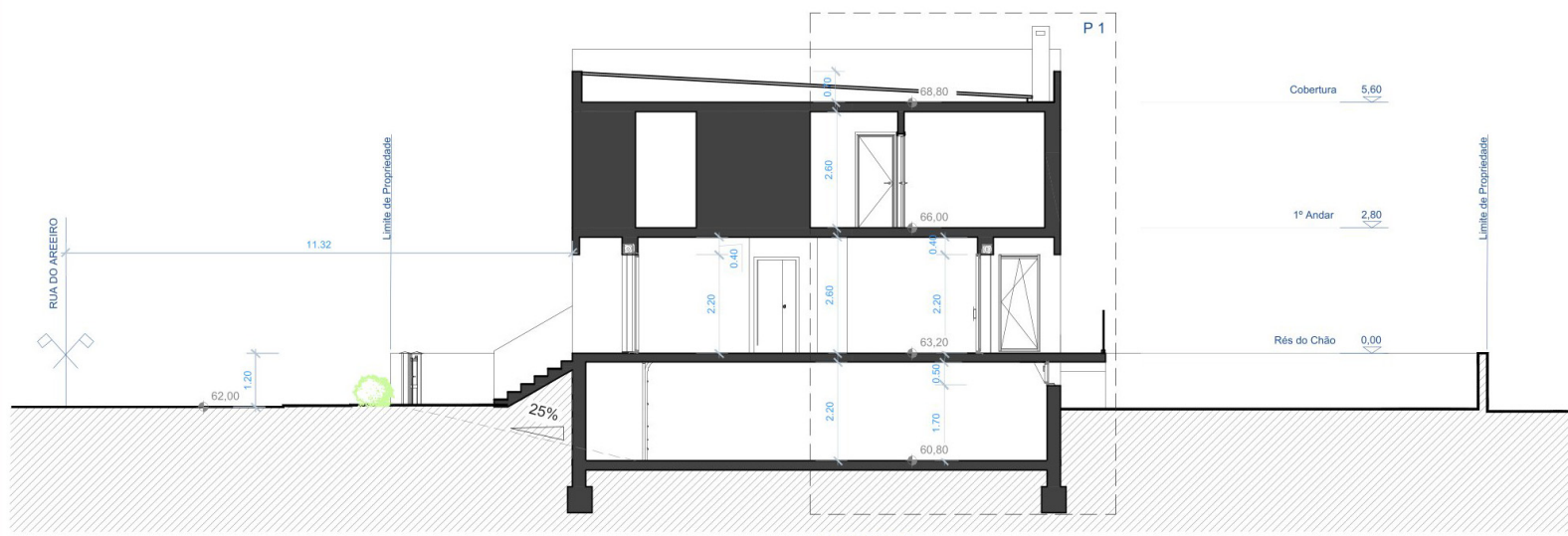
CORTE C-D
