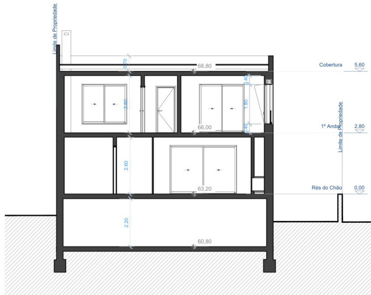
CORTE A-B
