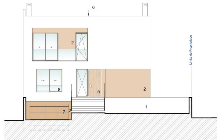
ALÇADO PRINCIPAL - NORTE
